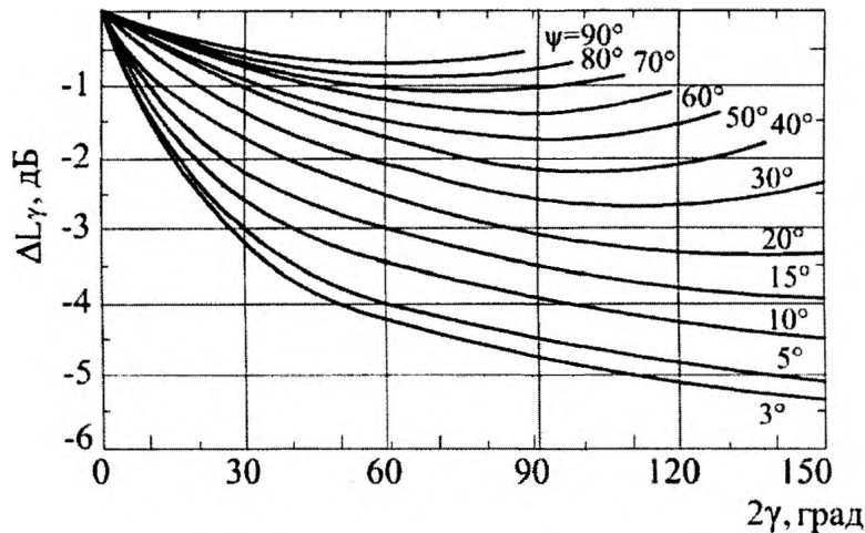
Рисунок 8 – Номограма для визначення величини поправки \Delta L_\gamma
