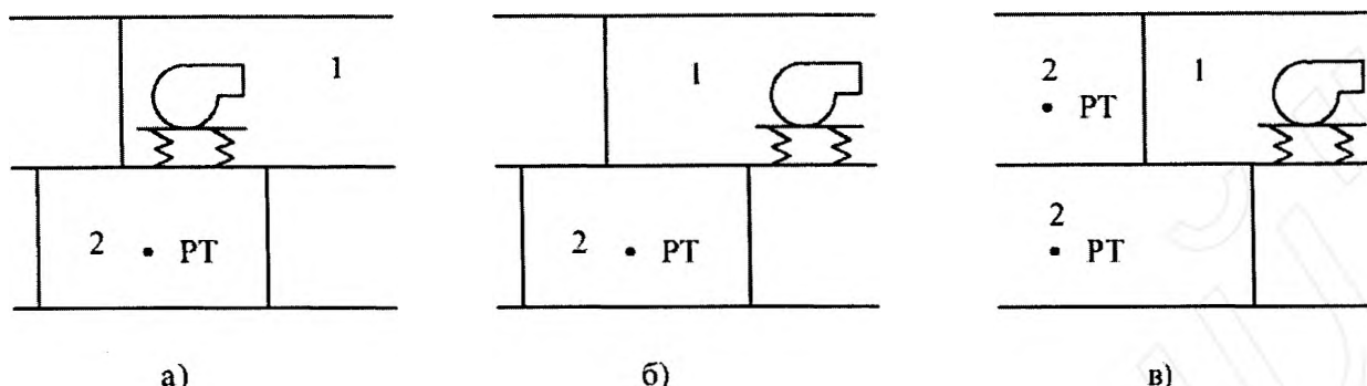
Рисунок Е.1 – Схеми взаємного розміщення приміщення з інженерним обладнанням і приміщень, що захищаються від шуму
