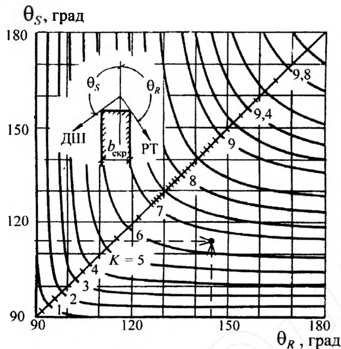
Рисунок 5 – Номограма для визначення коефіцієнта K_i у формулі (34)
