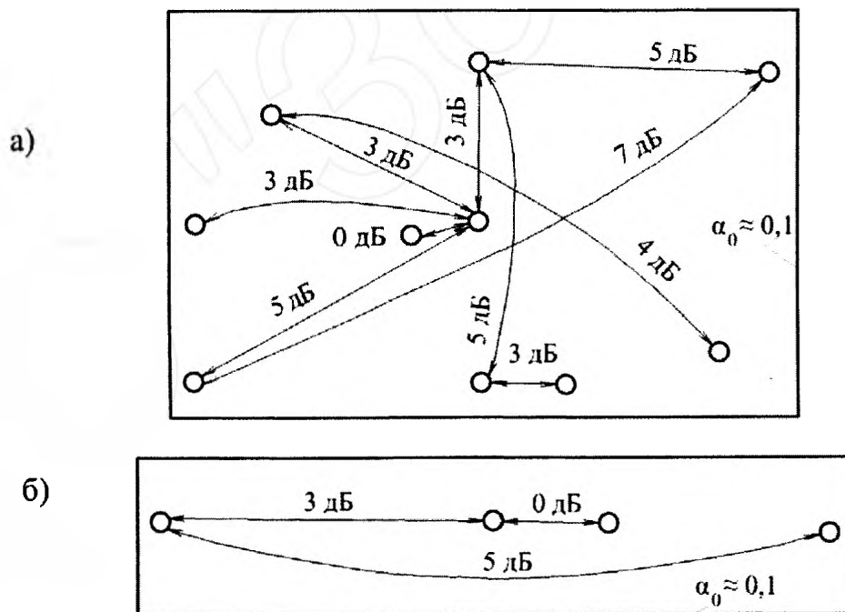
Рисунок 2 – Поправка \Delta L_{\text{відб}} для різних варіантів взаємного розташування джерела шуму і розрахункової точки в непропорційному необлицьованому приміщенні
